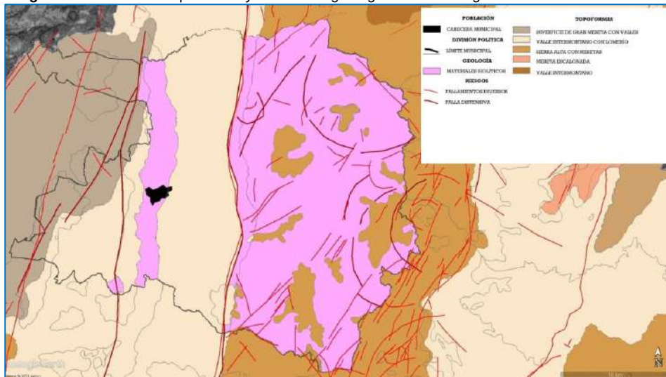
Imagen 6. Fallas contra topoformas y materiales geológicos. Tlaltenango.
