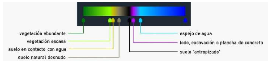
Figura 1. Escala de colores y clasificación especial del (UI) de Kawamura.
